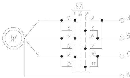
Рисунок 4.1 Электрическая схема лебедки JM, г/п 0,5-5т.
